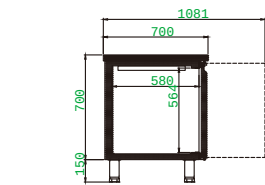
GN2100BT GN3100BT GN4100BT
