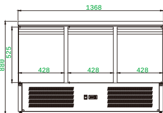
S903 S/S Top
