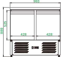
S901 S/S Top
